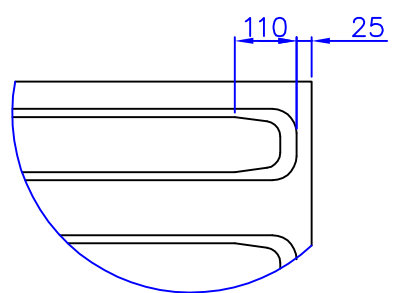
DETAIL B 2:1
