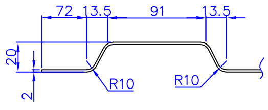
DETAIL C 2:1
