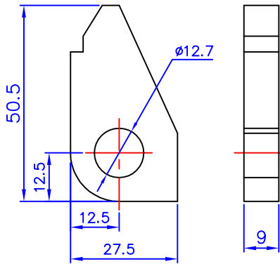
CIMC-D24-06 Hinge Lug 小吊耳 Material: SS400
